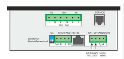
Fig.: Prophi® 7 interface
