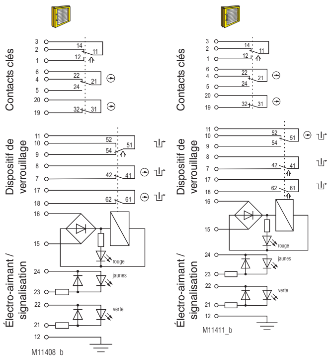
Fig. 1 : Gâche à l'état activé: Électro-aimant verrouillé, 1 re Clé à retirer, actionneur et 2 e clé insérés, porte fermée
