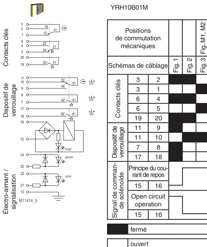
Fig. 3 : Verrouillage à l'état désactivé : Électro-aimant déverrouillé, Clé insérée
