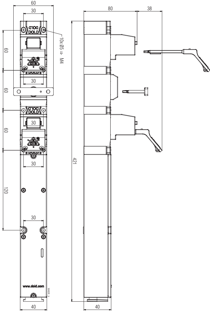
YRH10B01M Tolérances générales \pm 2\%
